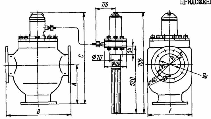
Габаритные размеры терморегуляторов РТПД-125, РТПД-150
