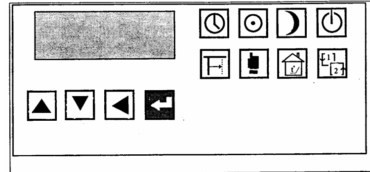
Рис. 3. Расположение функциональных кнопок на передней панели РТ.
