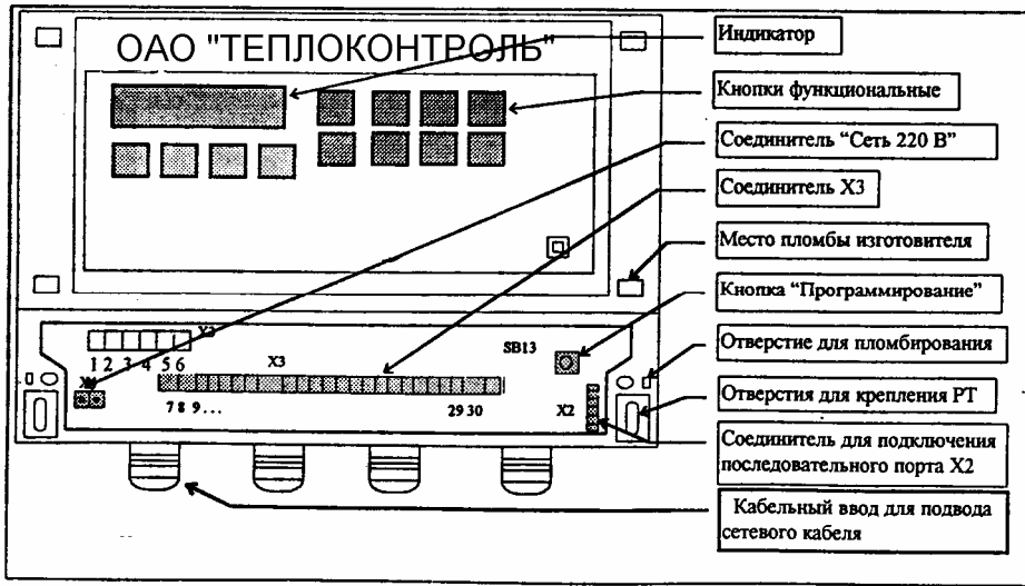
Рис. 1. Конструкция регулятора температуры.
